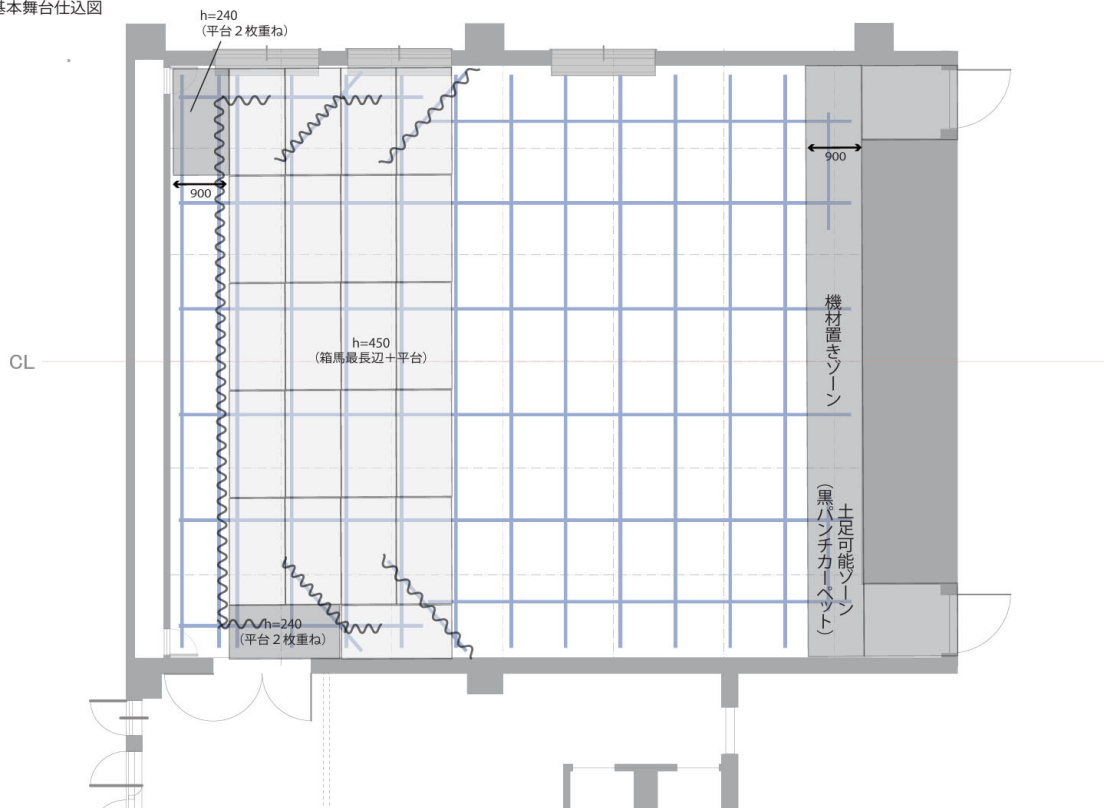
基本舞台仕込み図
