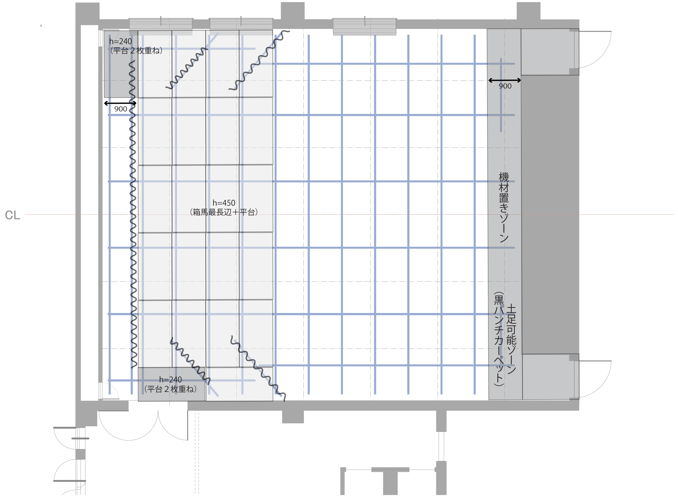
基本舞台仕込図
